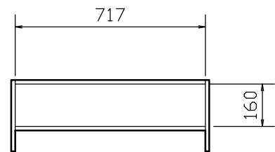
床部詳細図（底板なし）
