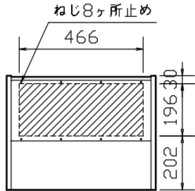
底板詳細図 斜線部 底板開口範囲 着脱底板 525×232×2.5t
